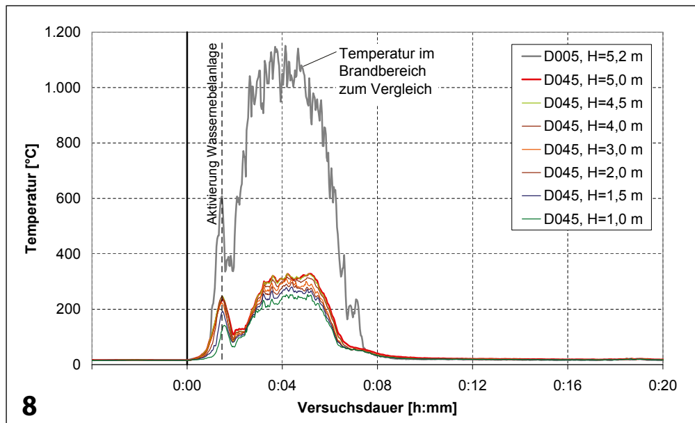
Temperaturen im Querschnitt 45 m hinter der Mitte der Brandlast (100 MW-Brand mit Wassernebel)
