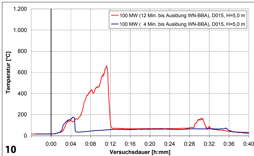
Temperaturverlauf unter der Zwischendecke 10 m hinter der Brandlast
