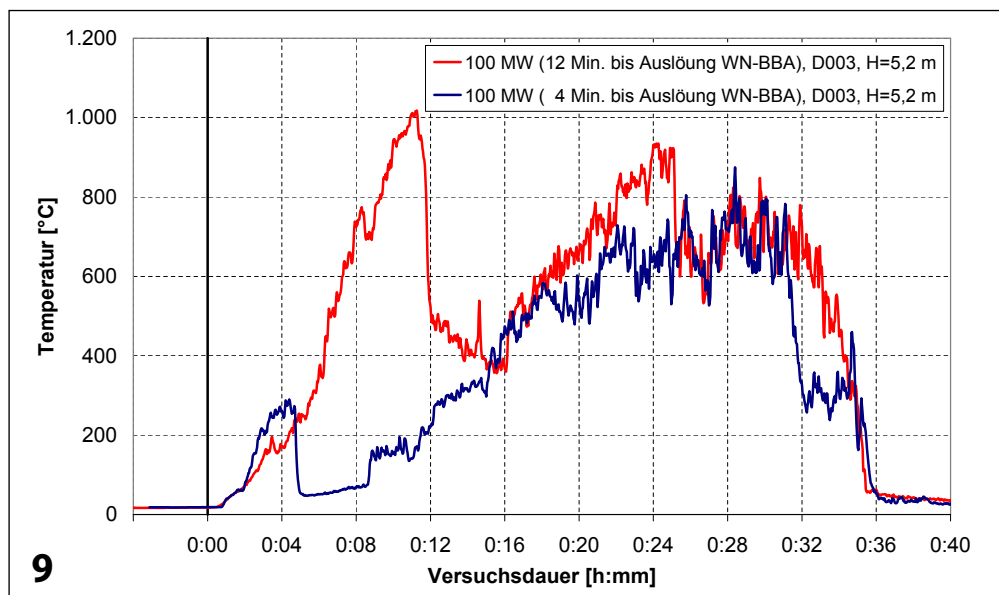
Temperaturen unter der Zwischendecke im Bereich der Brandlast (3 m hinter der Mitte der Brandlast)
